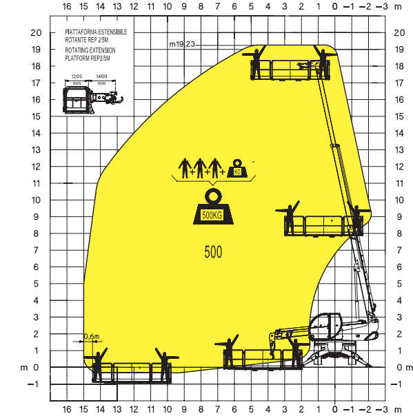
TP teleskopierbarer arbeitskorb mit 180° rotation
