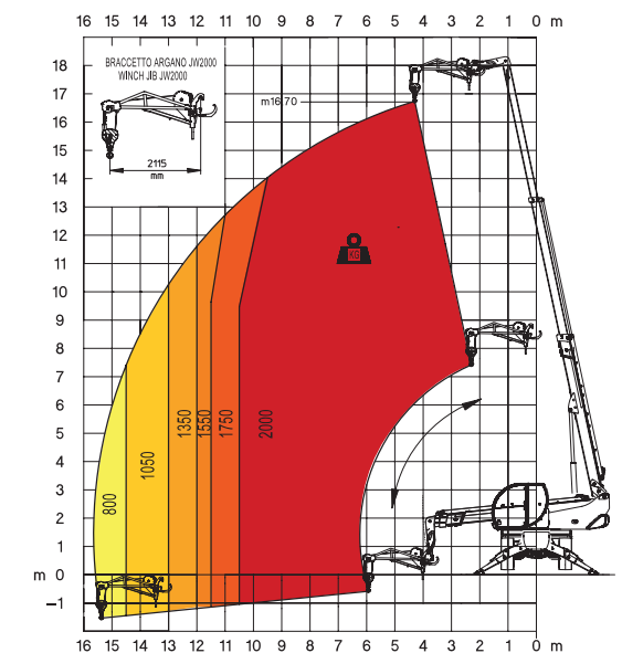
JW 2000 jib gittermastwinde 2.000
