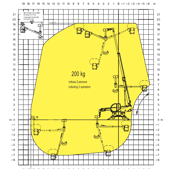
TP O-U teleskopierbarer arbeitskorb positiv-negativ mit 340° rotation
