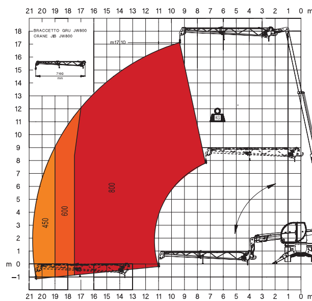
JW 800 jib gittermastwinde 800
