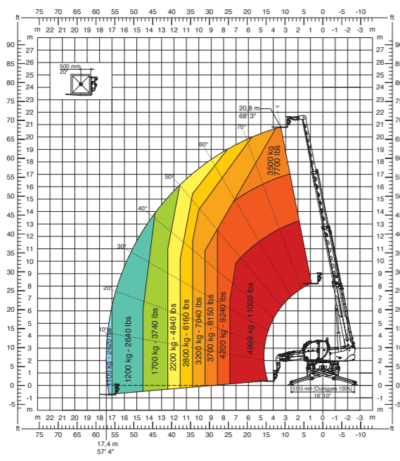
W 3,5 Lier 3,5 ton
