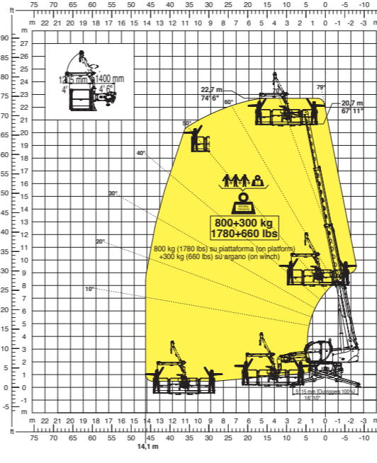
REP 8.2-4,7 WO,3 Werkplatform 4,7 m 800 kg met lier 300 kg
