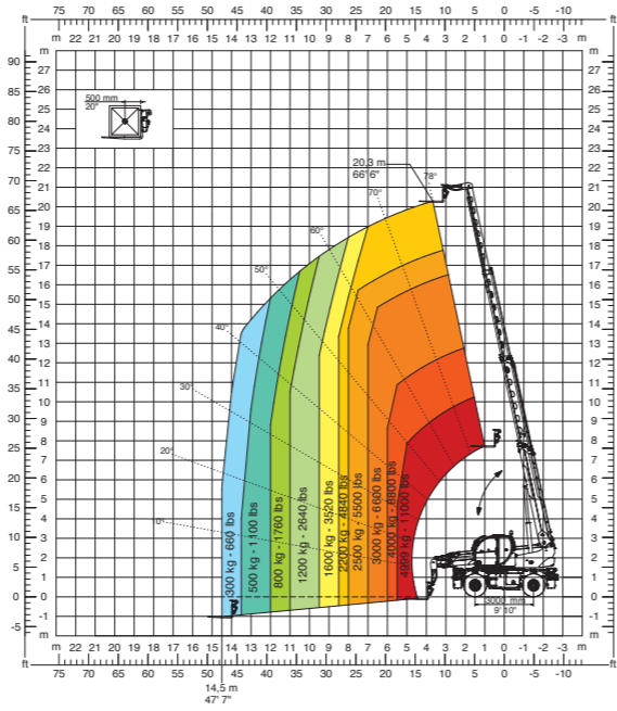
W 5 Lier 5 ton
