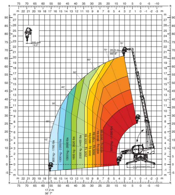
JW 2000 Jib lier 2.000 kg
